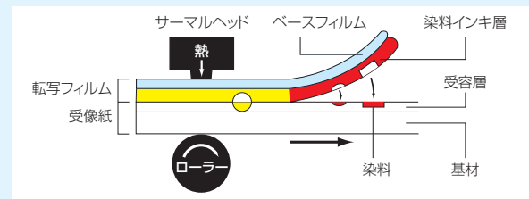
昇華型熱転写記録材の仕組み
